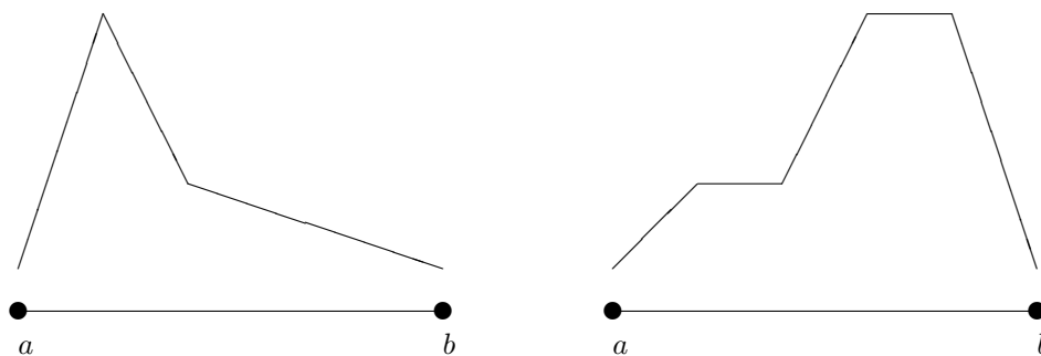
FIGURE 5. Quasi-concavité stricte et quasi-concavité
