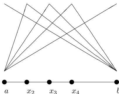
FIGURE 1. L'unimodalité de Black
